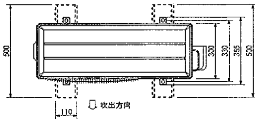
外観寸法図
